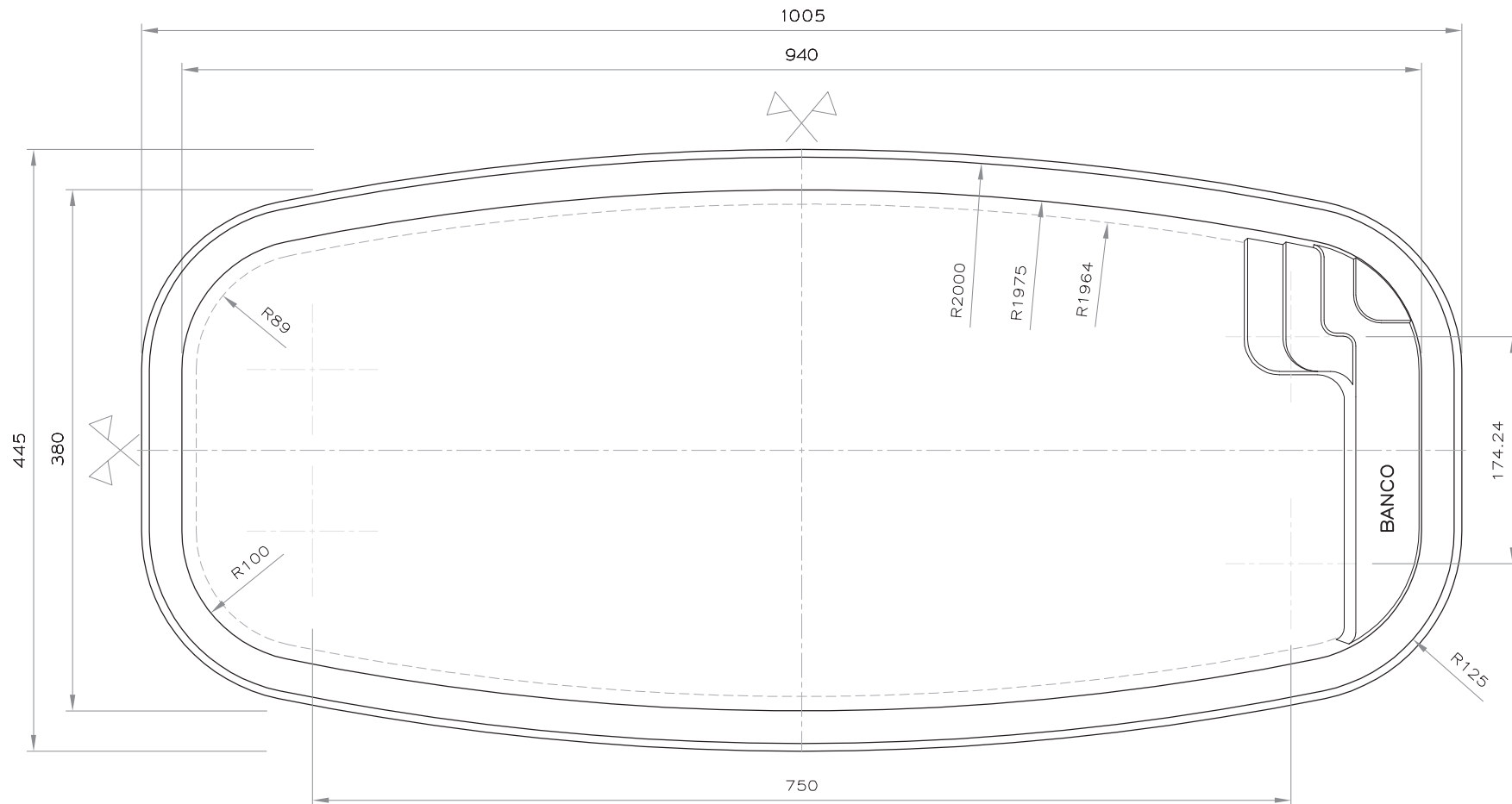
Vista Superior Escala 1/50
