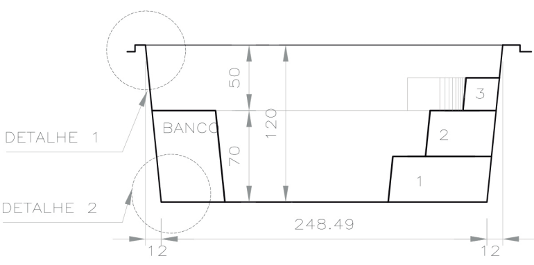
Corte Longitudinal Escala 1/40
