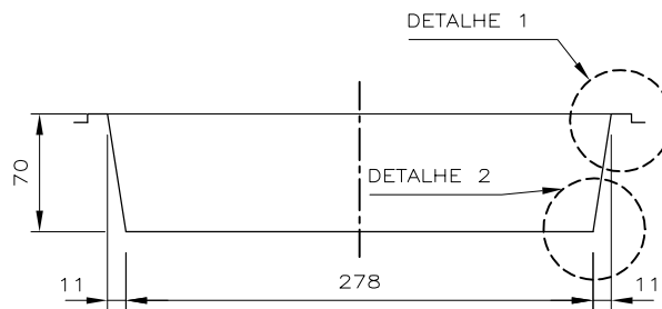
Corte Longitudinal Escala 1/50
