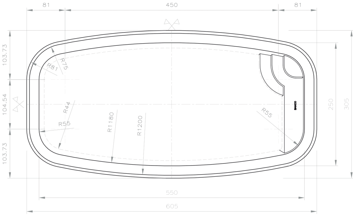
Vista Superior Escala 1/50
