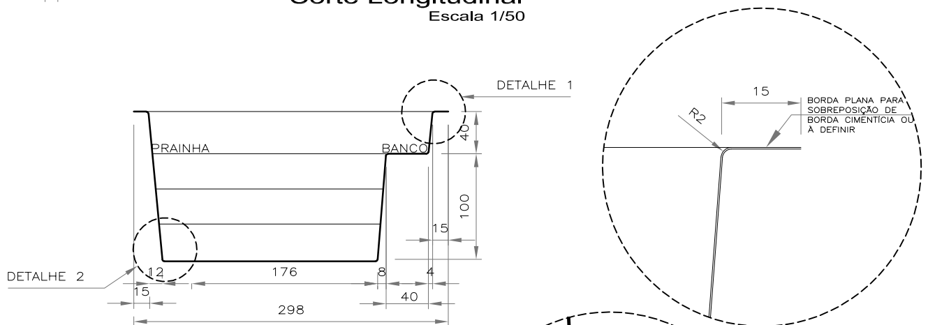
Detalhe 1 Escala 1/10
