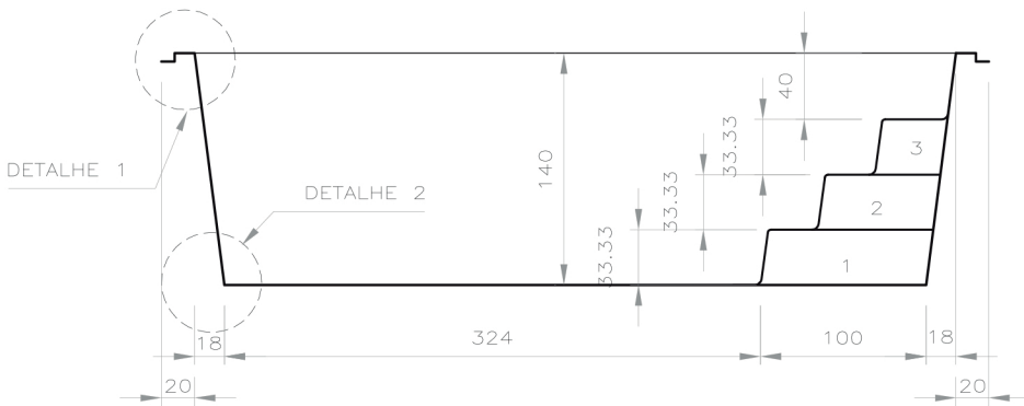
Corte Longitudinal Escala 1/50
