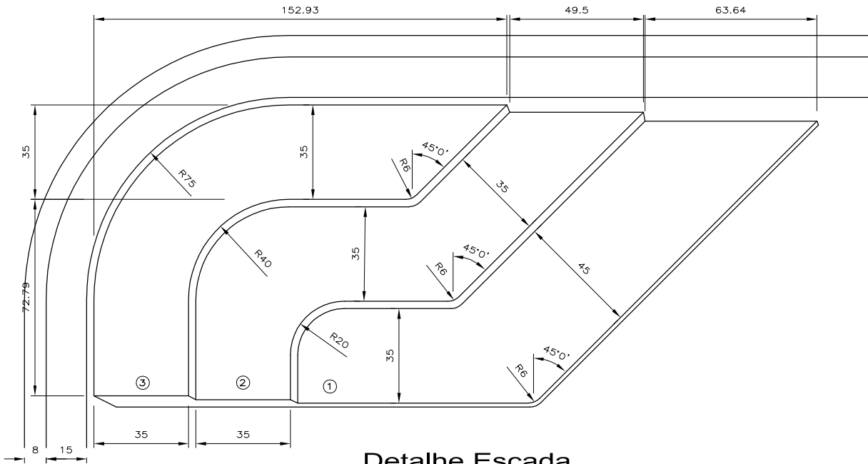
Detalhe Escada Escala 1/20
