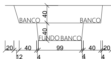
CORTE BB ESC 1:50
