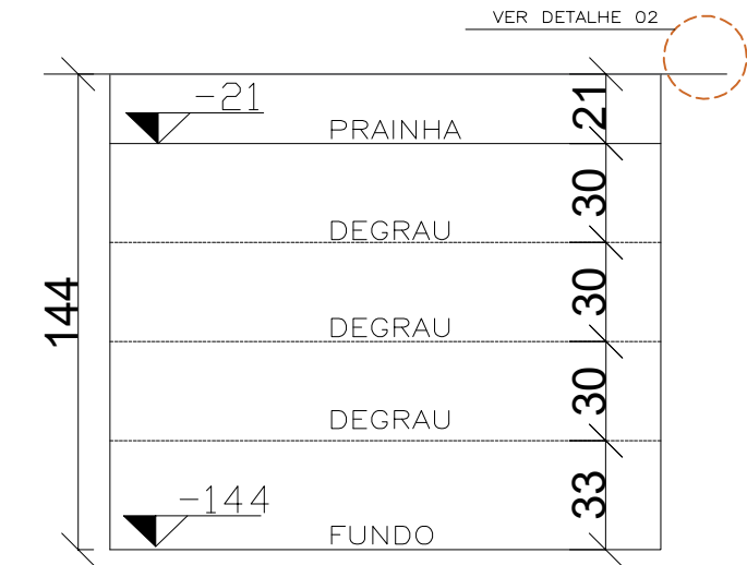
CORTE CC ESC 1:25
