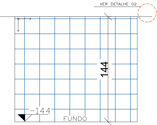
VISTA 03 ESC 1:25
