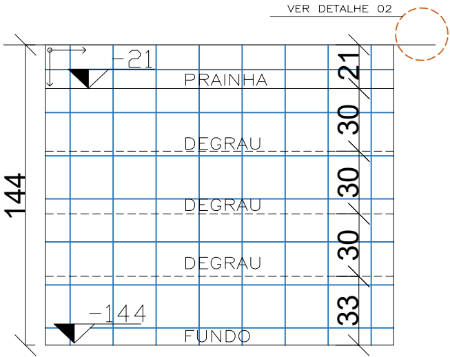
VISTA 04 ESC 1:25
