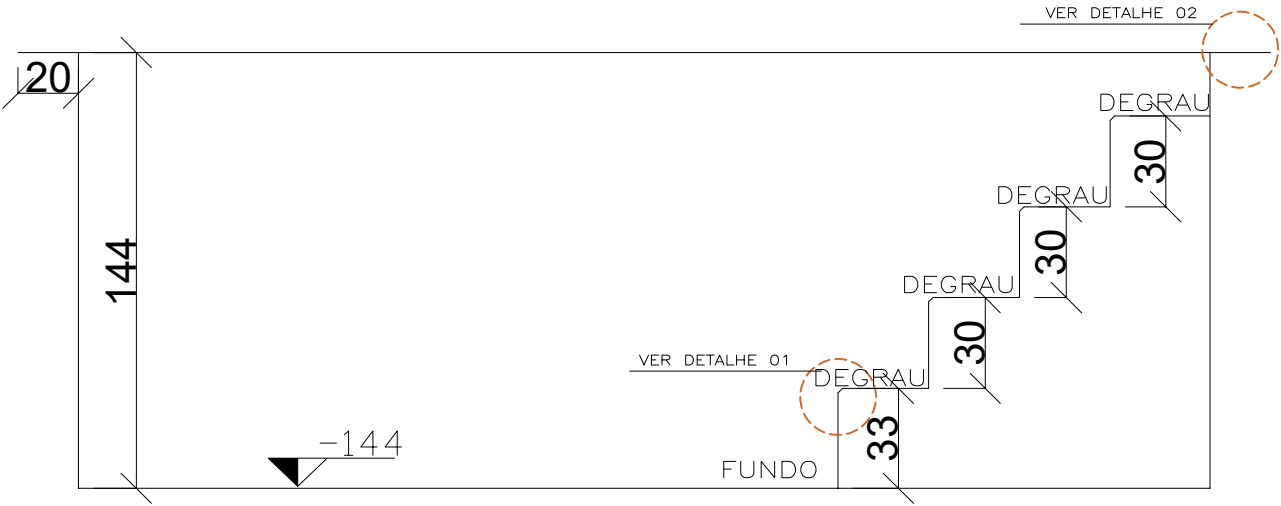
VISTA SUPERIOR ESC 1:40
