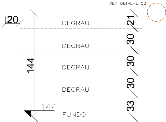
CORTE CC ESC 1:25
