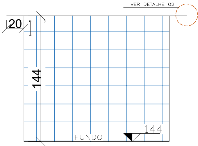
VISTA 03 ESC 1:25
