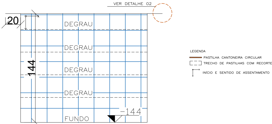
VISTA 04 ESC 1:25
