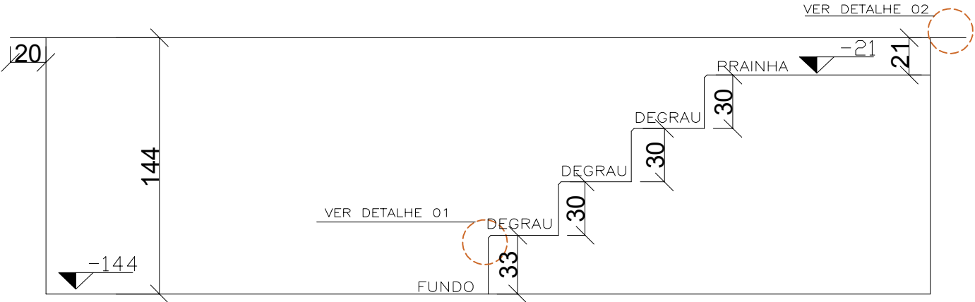
CORTE AA ESC 1:30
