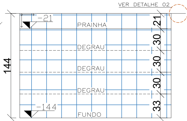
VISTA 04 ESC 1:25
