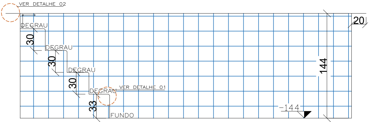
VISTA 02 ESC 1:30
