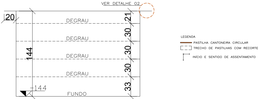
VISTA 04 ESC 1:30
