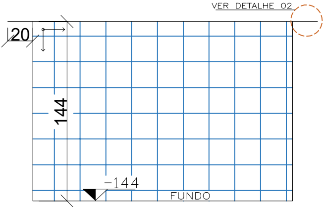
VISTA 03 ESC 1:30
