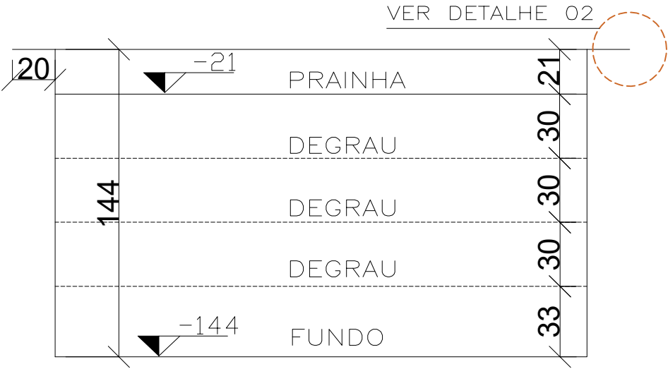
CORTE CC ESC 1:25
