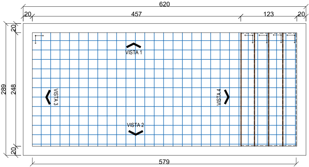
VISTA SUPERIOR ESC 1:50
