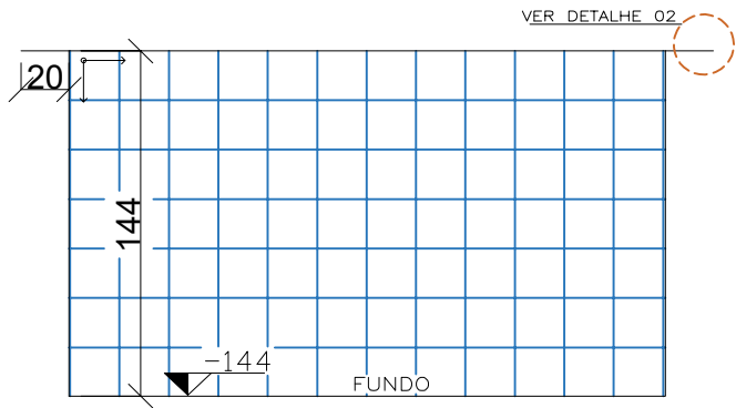
VISTA 03 ESC 1:35
