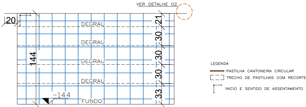
VISTA 04 ESC 1:35
