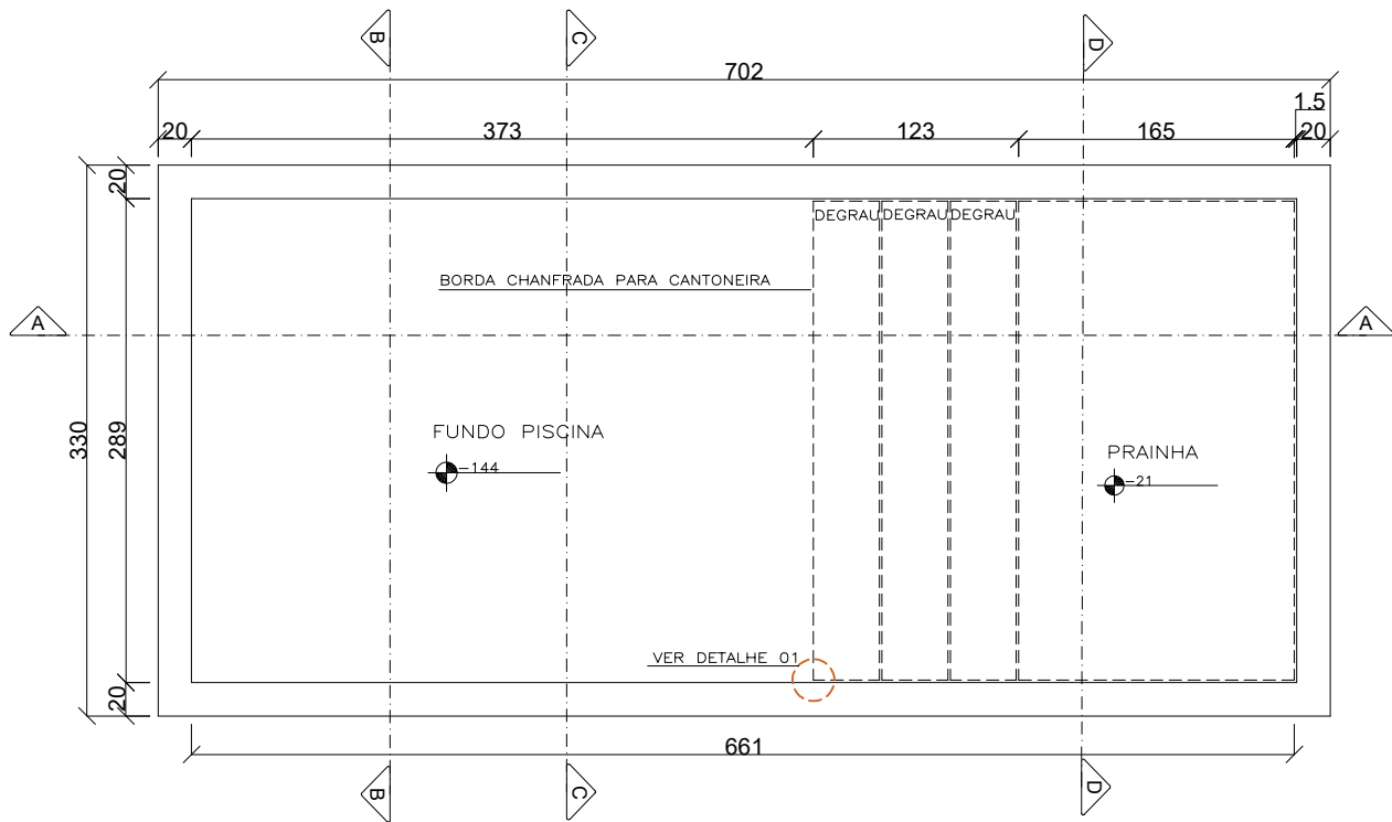
VISTA SUPERIOR ESC 1:50
