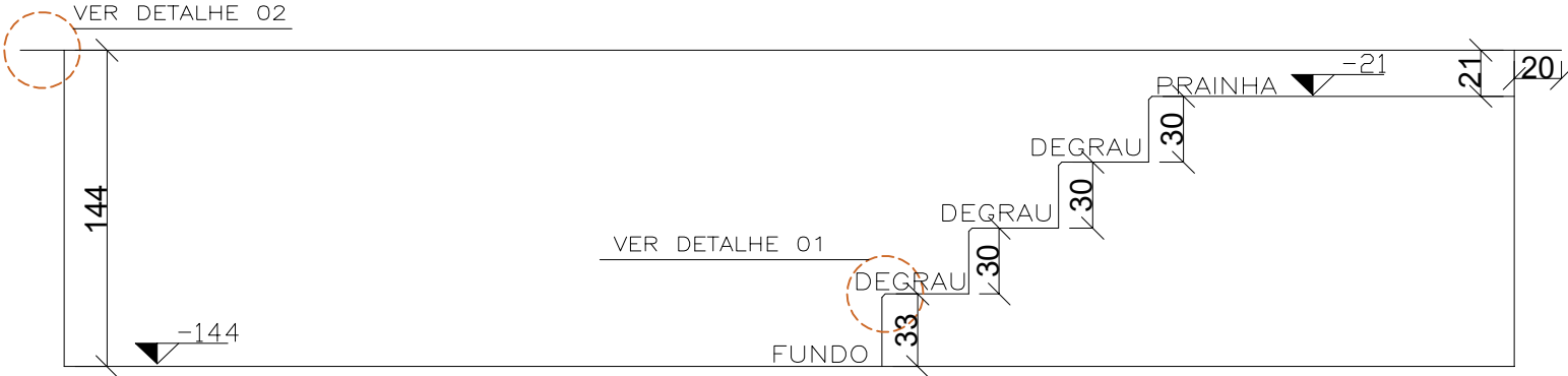
CORTE AA ESC 1:35
