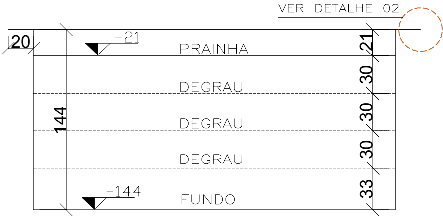
CORTE CC ESC 1:30
