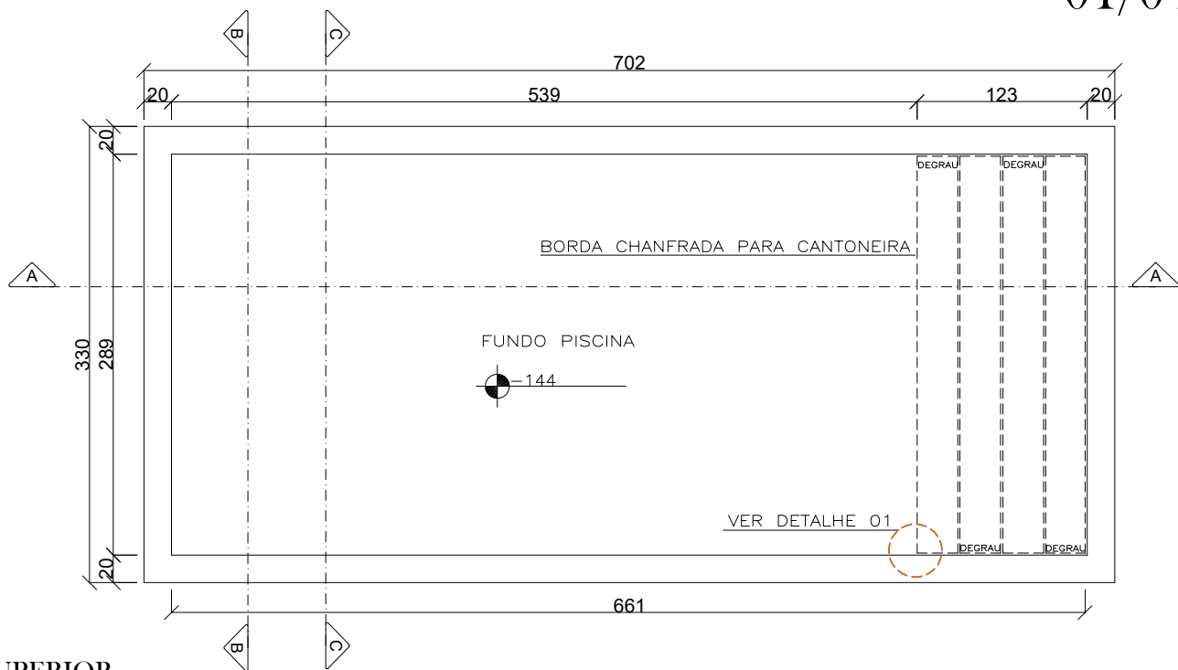
VISTA SUPERIOR ESC 1:50
