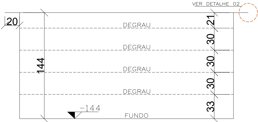
CORTE CC ESC 1:25
