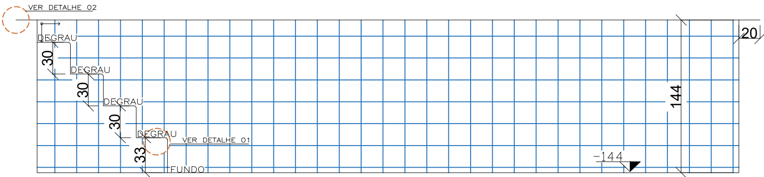
VISTA 02 ESC 1:35
