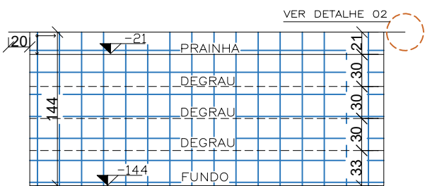
VISTA 04 ESC 1:50
