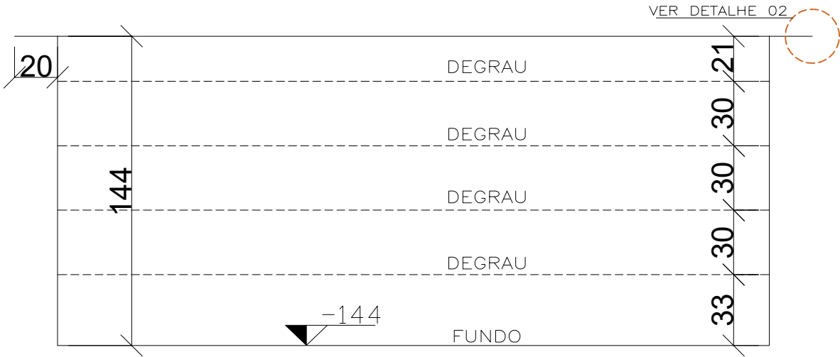
CORTE CC ESC 1:25
